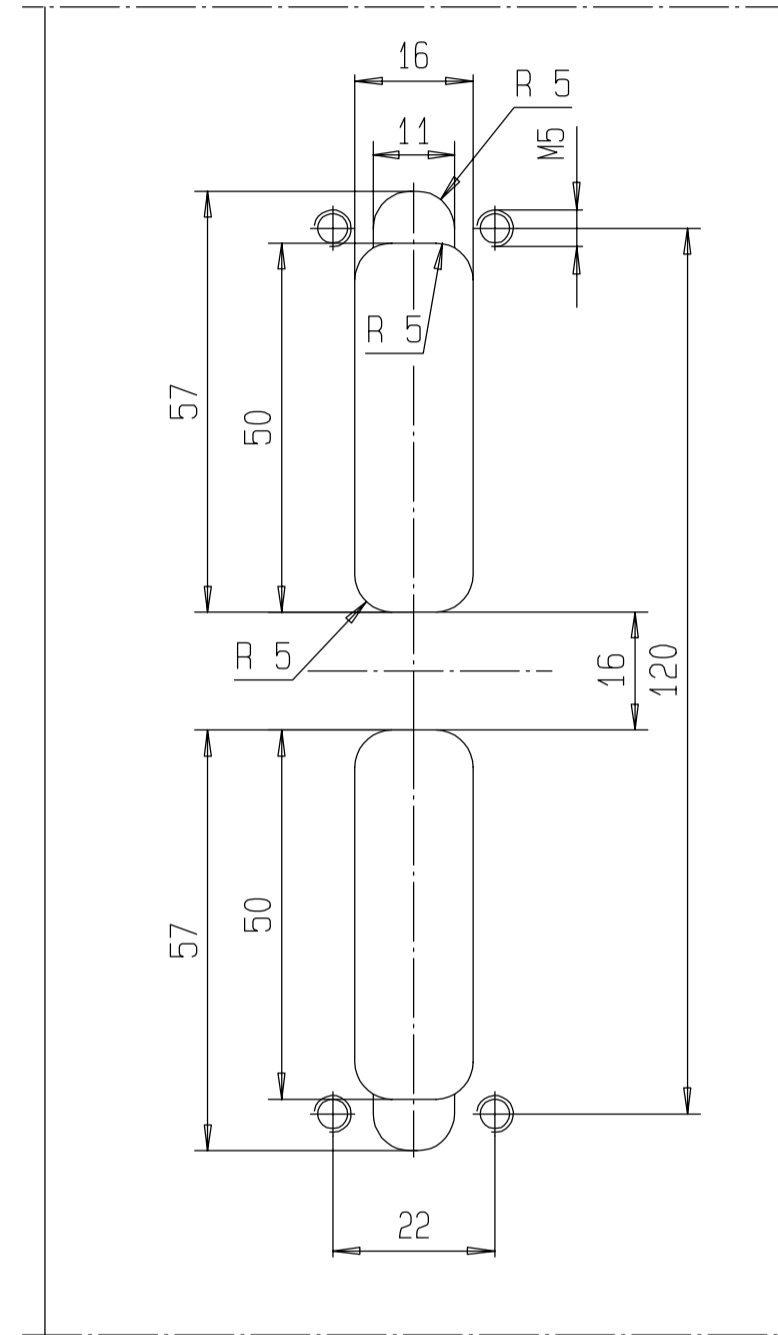
Fräsung bei Verwendung der Gewindeansätze ZA02DV
