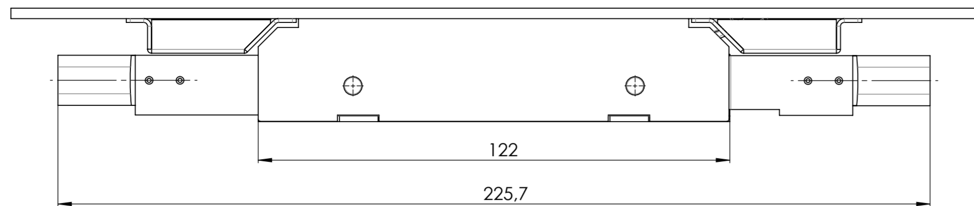
Darstellung verriegelt
