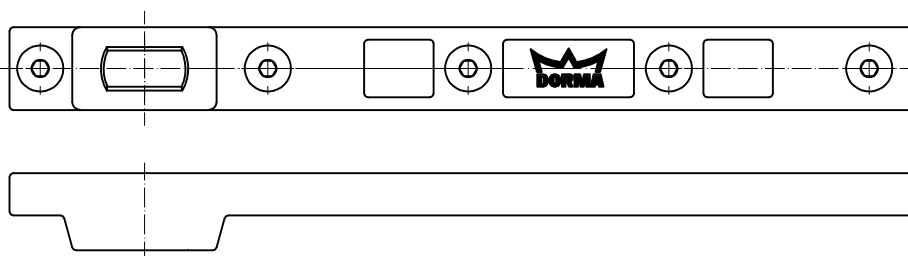
Unterer Stahlrührheber (nur mit BTS) Art. Nr.: 04.605
