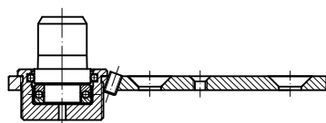
Bodenlager Art. Nr.: 01.106
