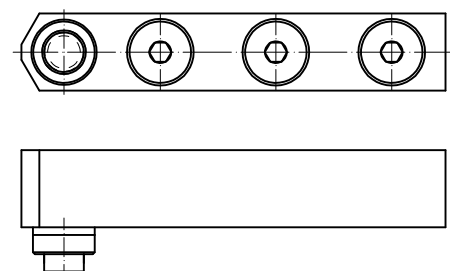
Unteres Zapfenband Art. Nr.: 804.060.002.50
