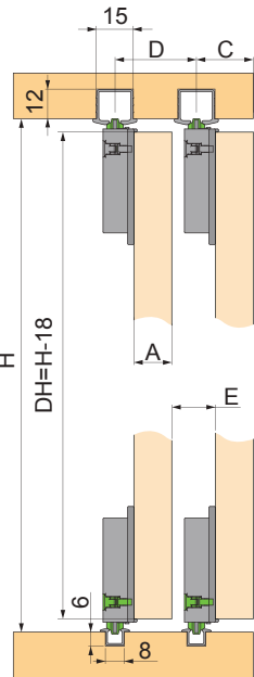
Beidseitige Dämpfung Both sides damping
