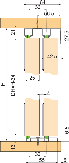
Beidseitige Dämpfung Both sides damping
