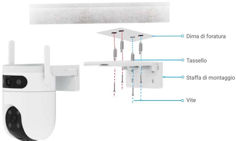
Fig. 1 Montaggio a soffitto
