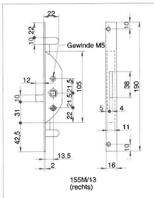
Einstecktrieb mit Stulp 155M/13
