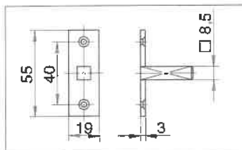
Träger mit Vierkantstift 293
