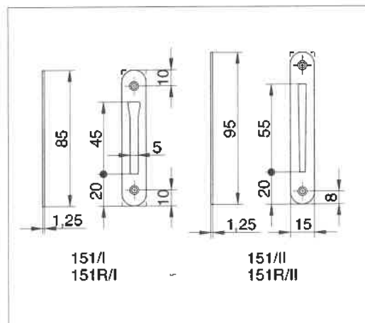
Schließbleche für Einstemmungen 151
