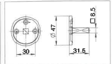
Rosettenträger 293TR
