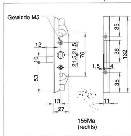
Einstecktrieb ohne Stulp 155Ma
