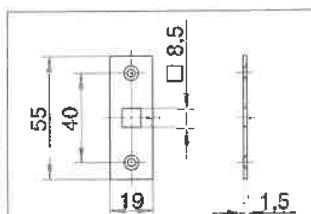
Fixierplättchen 292
