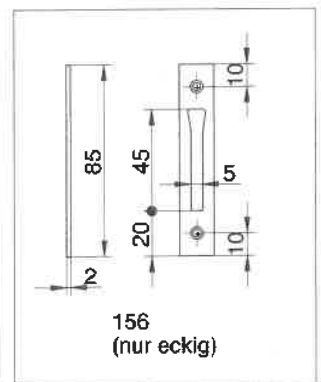
Schließblech 156
