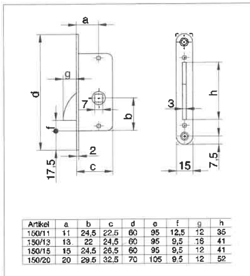
Einstemmungen + Schließblech 150
