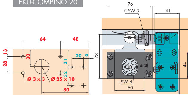
EKU-COMBINO 20
