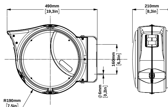
dimensioni AM85
